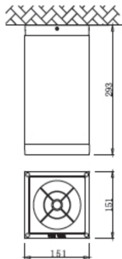
金卤光源灯具尺寸图
